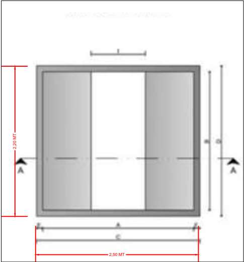
PIANTA TIPO TOMBA DI FAMIGLIA A 8 POSTI
