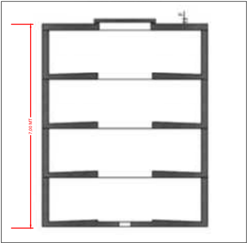
SEZIONE TIPO TOMBA DI FAMIGLIA A 8 POSTI
